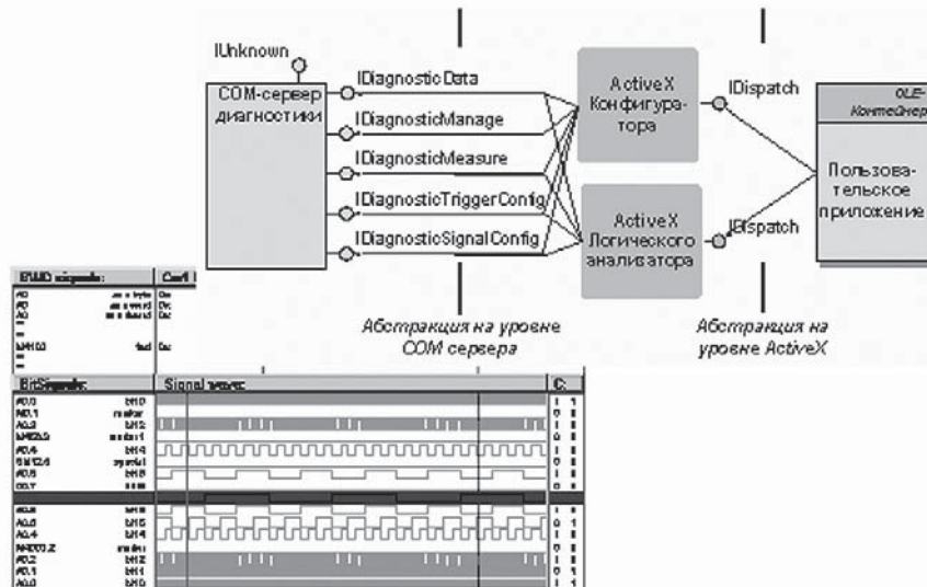
Рис. 2. Логический анализатор
