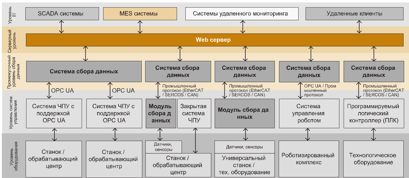
Рис. 1. Варианты взаимодействия системы сбора данных с разнородным технологическим оборудованием в рамках производственного участка
