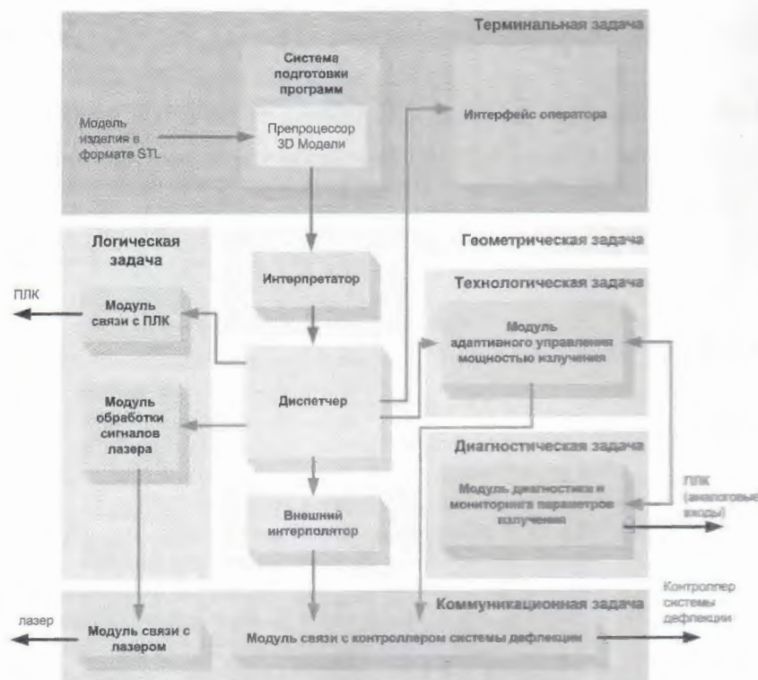
Рис. 2. Модульная структура системы управления установкой лазерного синтеза
